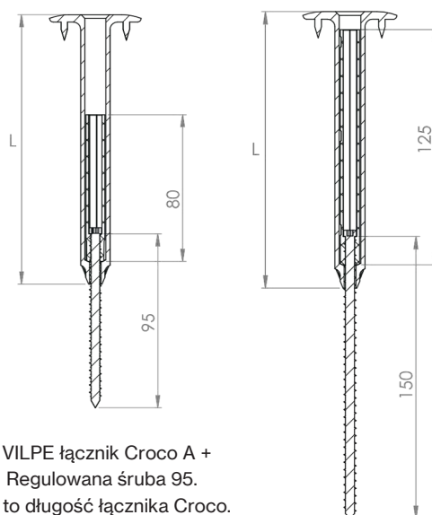
VILPE łącznik Croco A + Regulowana śruba 150. L to długość łącznika Croco.
